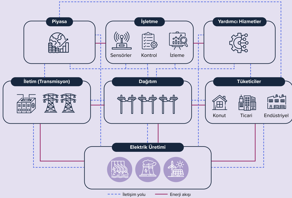
Şekil 12. Akıllı Şebeke Kavramsal Modeli: Enerji Akışı ve Haberleşme Yolları
