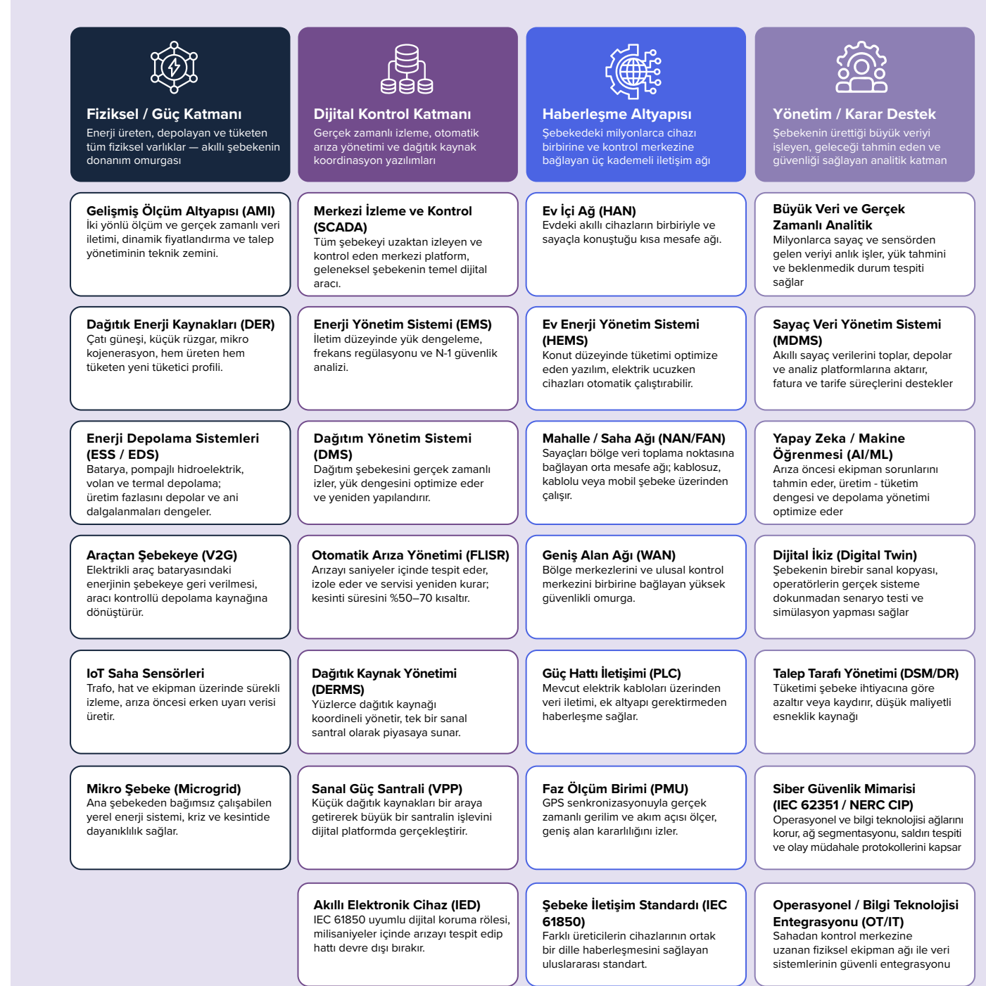
Şekil 9. Akıllı Şebekenin Katman Bazlı Bileşenleri
