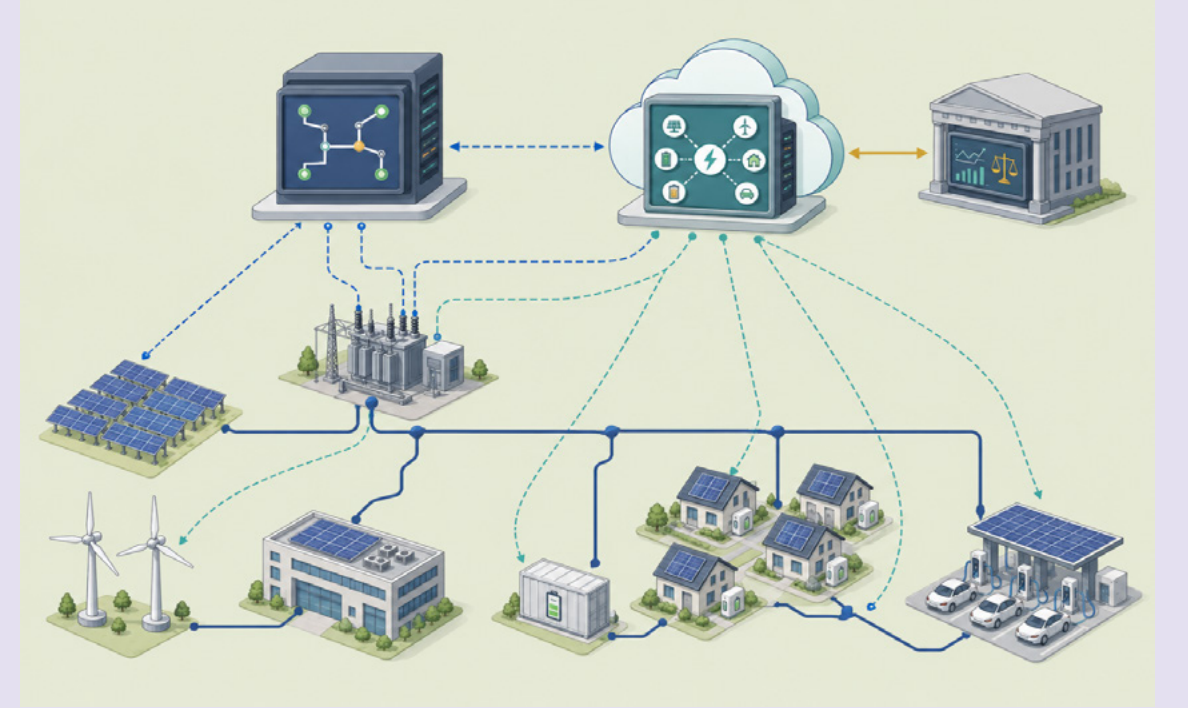
Şekil 14. DERMS ve Sanal Güç Santrali Aracılığıyla Dağıtık Enerji Kaynaklarının Teknik ve Piyasa Odaklı Koordinasyonu
