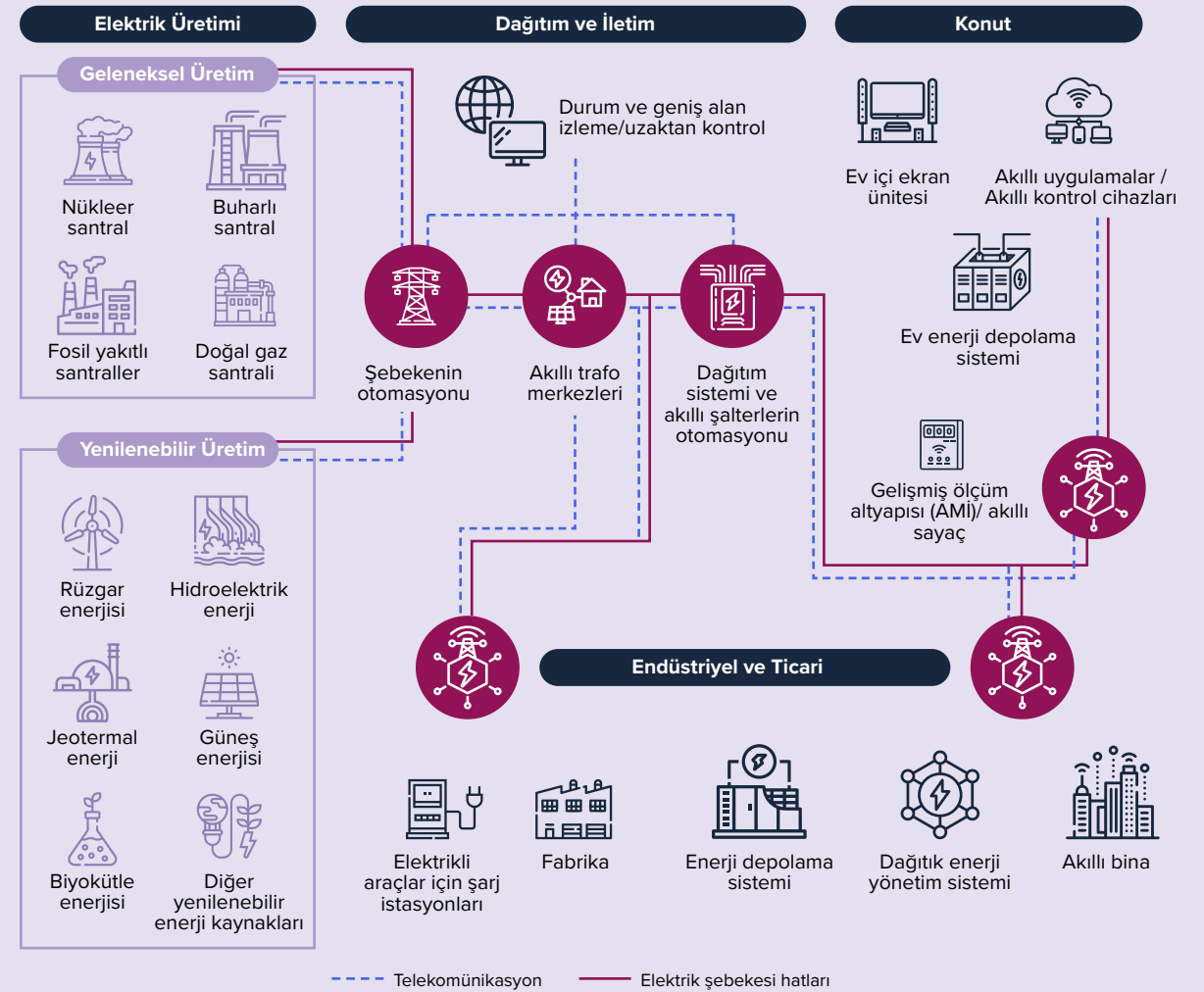
Şekil 7. Akıllı Şebeke Mimarisi
