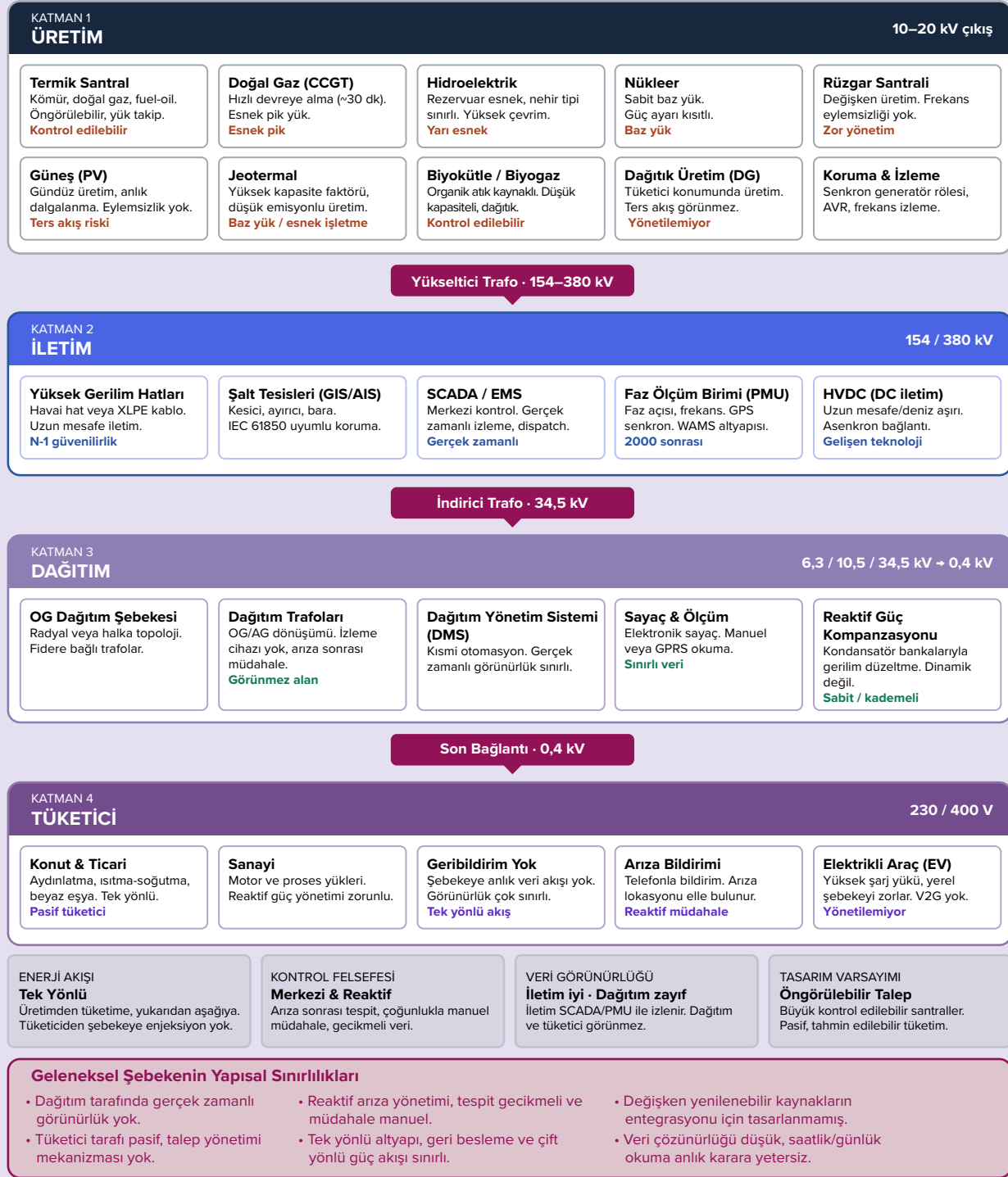
Şekil 2. Geleneksel Şebekenin Üretim–İletim–Dağıtım–Tüketim Hiyerarşisi
