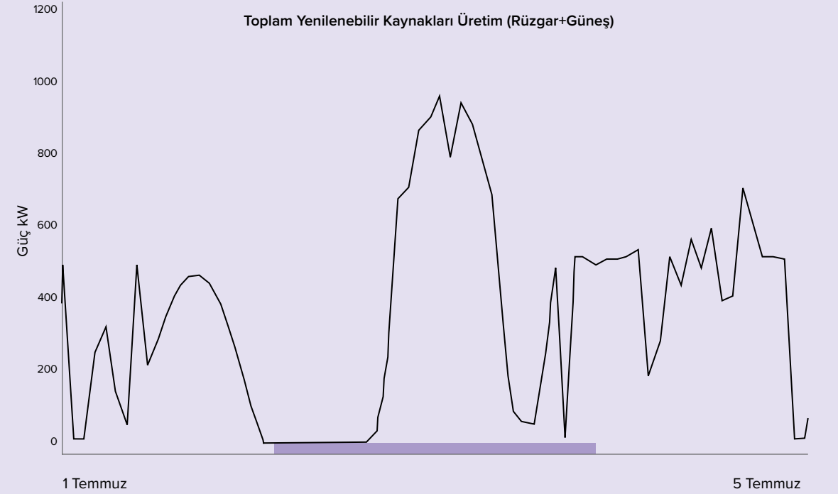
Şekil 6. Yenilenebilir Kaynaklarının (Rüzgar + Güneş) Değişken Üretim Profili
